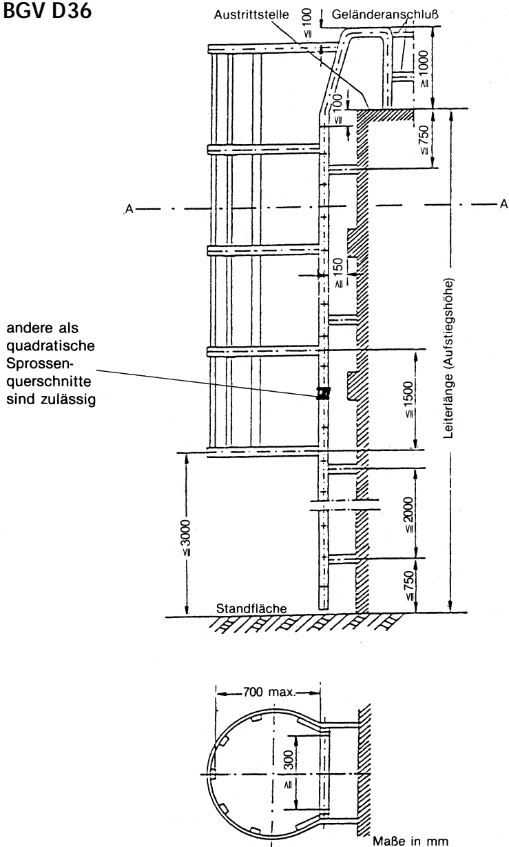
Bild 5: Steigleiter mit Rückenschutz
