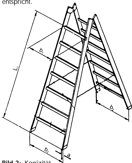
Bild 3: Konizität
